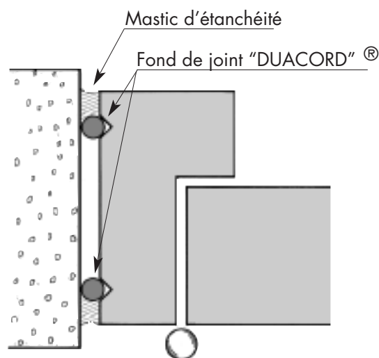
Fond de joint "DUACORD"® entre tableaux.
