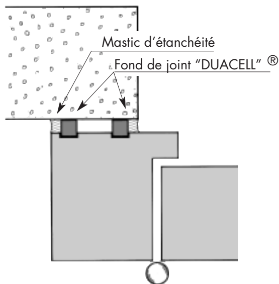
Fond de joint "DUACELL"® en applique.
